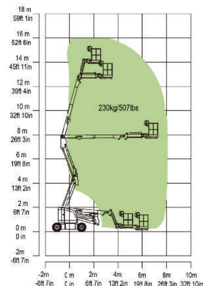
Curva de amplitud de plataforma ZA14JE
