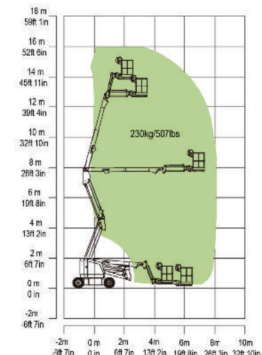
Curva de amplitud de plataforma ZA14JE-Li
